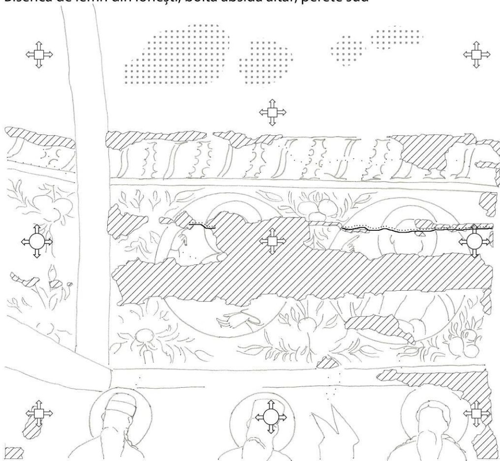
Biserica de lemn din Ionești, boltă absidă altar, perete sud
